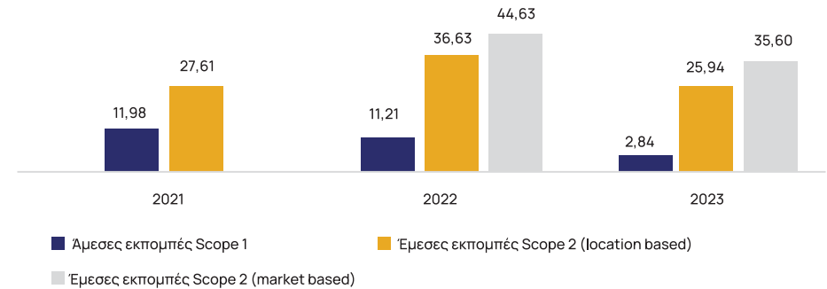
Γράφημα 4: Ετήσιες εκπομπές ΑτΘ (tCO 2 e /εργαζόμενο)
