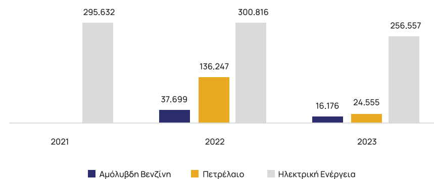
Γράφημα 2: Κατανάλωση ενέργειας (MJ)
