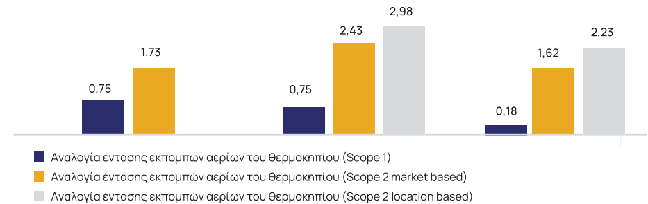
Γράφημα 5: Ένταση εκπομπών ΑτΘ (tCO 2 e /εργαζόμενο)
